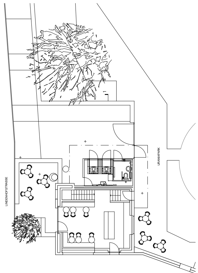
Grundriss EG
